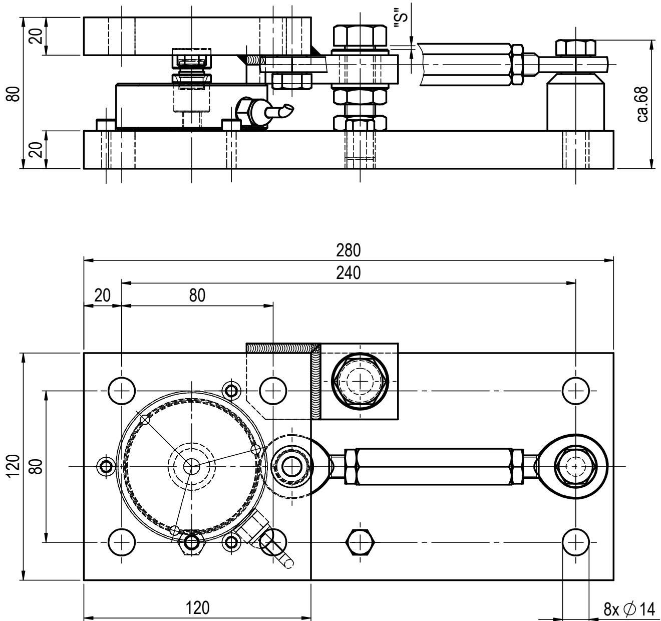
Anordnung der Lastecken gemäß Schema 550-04-01-4
